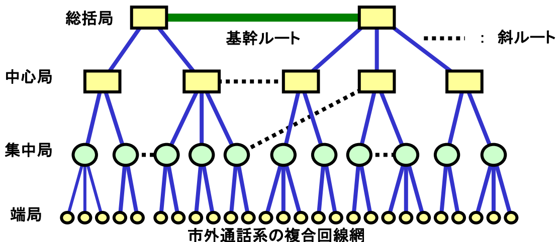
図 2-22 電話交換網の構成
